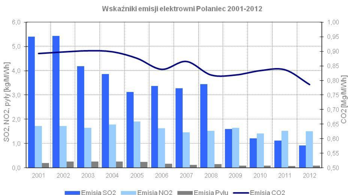
Rys. 1 Wskaźniki emisji elektrowni Połaniec w latach 2001 – 2012
